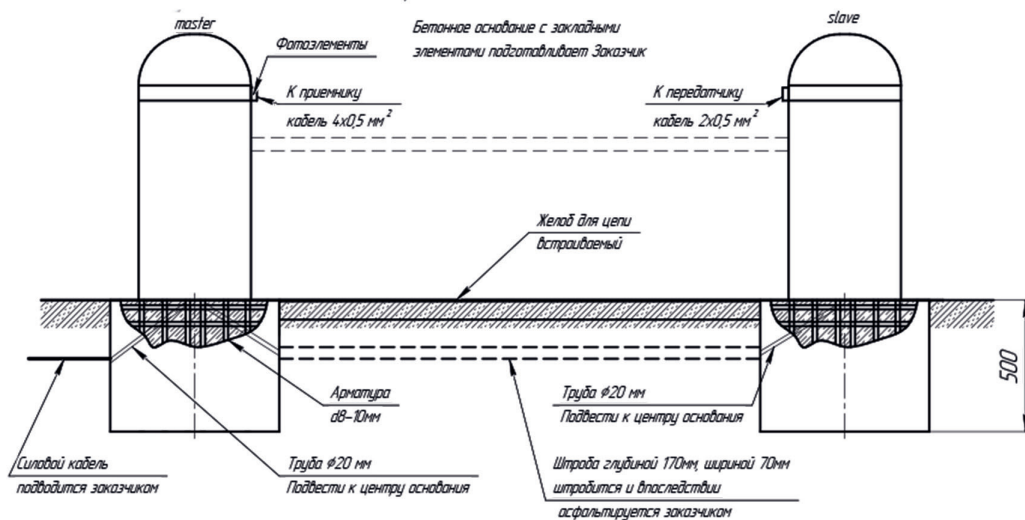
Схема электроподготовки и подготовки основания
