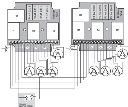
Рис. 3. Схема соединений блоков GC4
