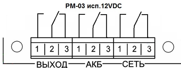
Рисунок 3. Переключающий контакт, выведенный на клеммы выходных колодок модуля
