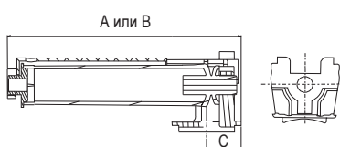
Для крепления Арт. № 9162135
