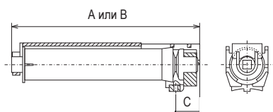
Для стандартного крепления
