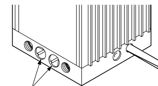
Перепускные винты
