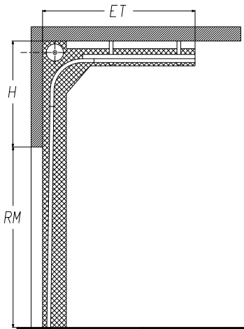
Высокий тип монтажа с верхним расположением вала
