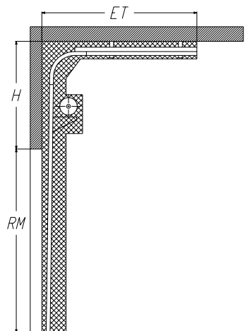
Высокий тип монтажа с нижним расположением вала
