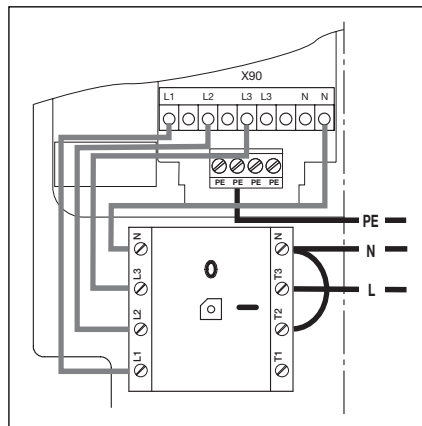
4-6.3 Тип двигателя K09WS: провод для подключения сети однофазного переменного тока к главному выключателю не должен быть скручен!
