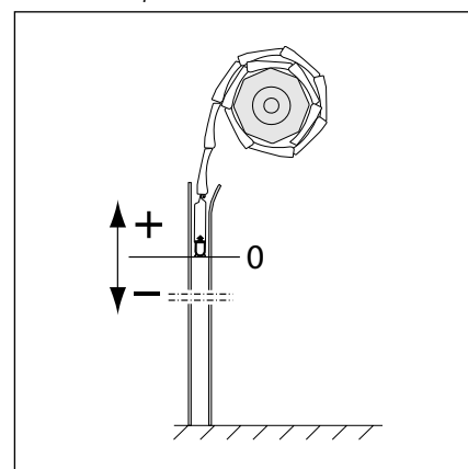
6-5.2 Направление движения для тонкой регулировки -Конечное открытое положение ворот-
