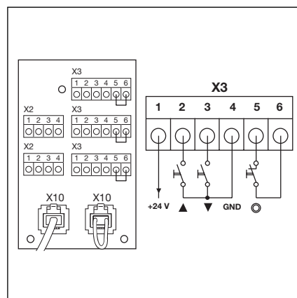
4-4.2 Подключение дополнительных внешних элементов управления к X10
