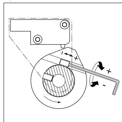
6-5.3 тонкая регулировка неподвижного контактного кулачка S3 -Конечное открытое положение ворот-
