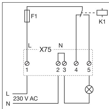
7-4.4 Схема реле и пример подключения для лампы на 230 В
