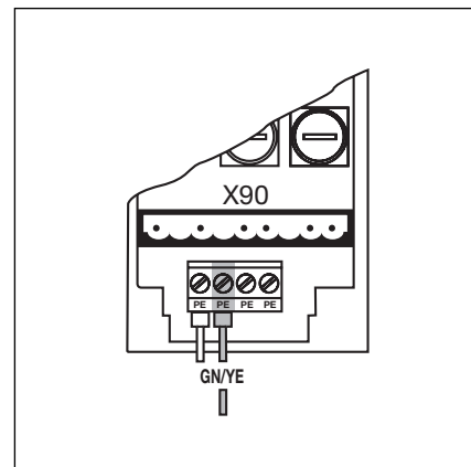
4-5.4 Подсоединение защитного провода кабеля для подключения к сети
