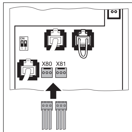
4-4.3 Подсоединение релейных плат к гнездам X80/X81
