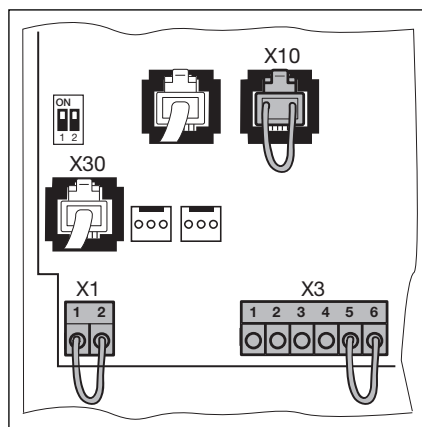
4-6.4 Вставные перемычки X1/X3, вставная перемычка X10
