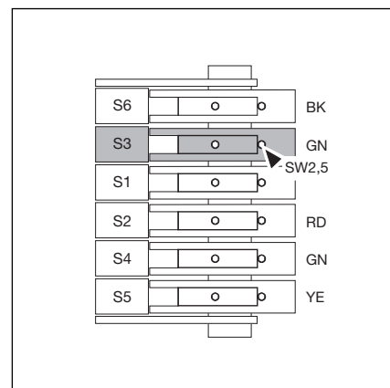
6-5.1 тонкая регулировка неподвижного контактного кулачка S3 -Конечное открытое положение ворот-
