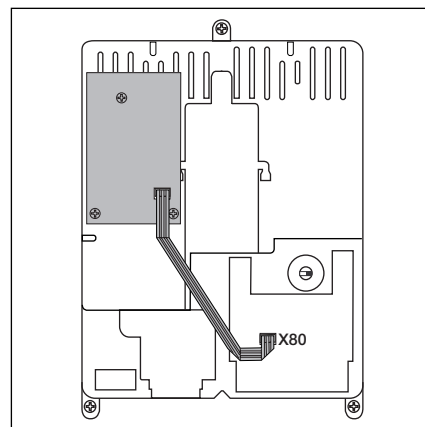
7-1.3 Монтаж платы расширения по ширине делительного модуля в корпусе системы управления и ввод кабеля для X80.
