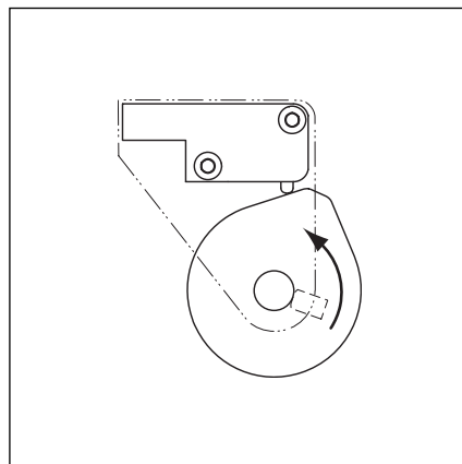
6-2.4 Направление движения коммутационного кулачка S3 - конечное положение закрытых ворот.
