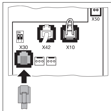
4-4.1 Подсоединение системных проводов, например, защитных устройств, к гнезду X30
