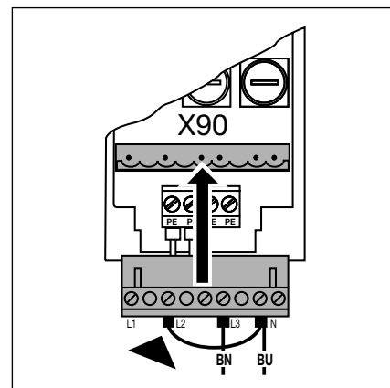
4-5.7 Тип двигателя K09WS: провод для подключения сети однофазного переменного тока к гнезду X90 не должен быть скручен!
