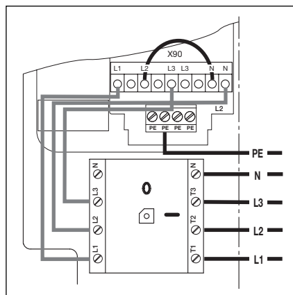
4-6.4 Подключение трехфазного переменного тока низкого напряжения без нулевого провода
