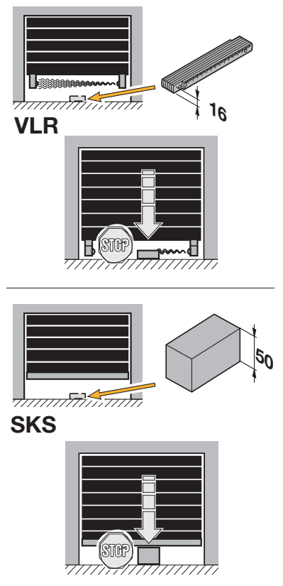
6-3.2 Проверка остановки по сигналу SKS
