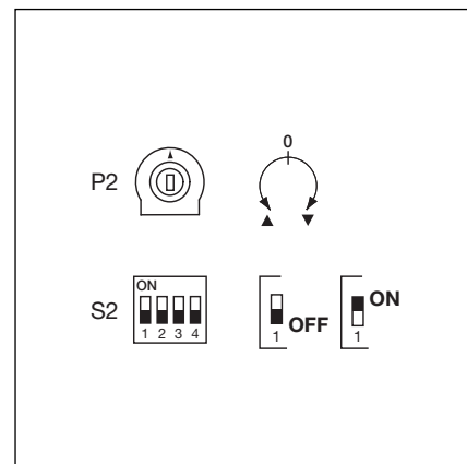
6-1.2 Потенциометр P2, DIL-выключатель S2 на плате управления
