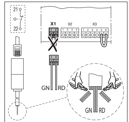
4-5.2 Подключение нормально замкнутой цепи X1
