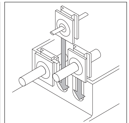
4-1.3 Установите резьбовое соединение кабеля
