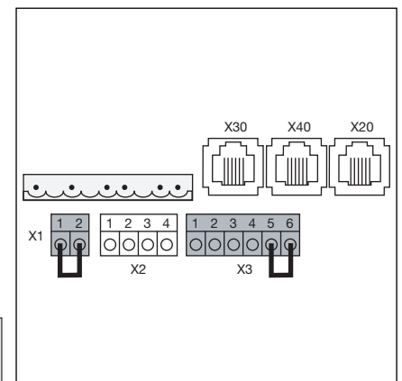
4-7.3 Штекерные перемычки X1 / X3
