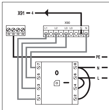
4-6.9 Подключение однофазной сети к главному выключателю
