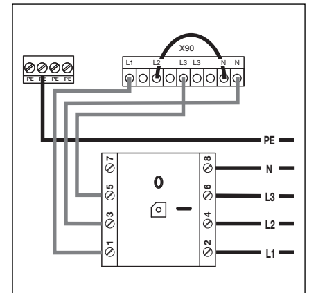
4-7.2 Подключение трехфазного переменного тока низкого напряжения без нулевого провода
