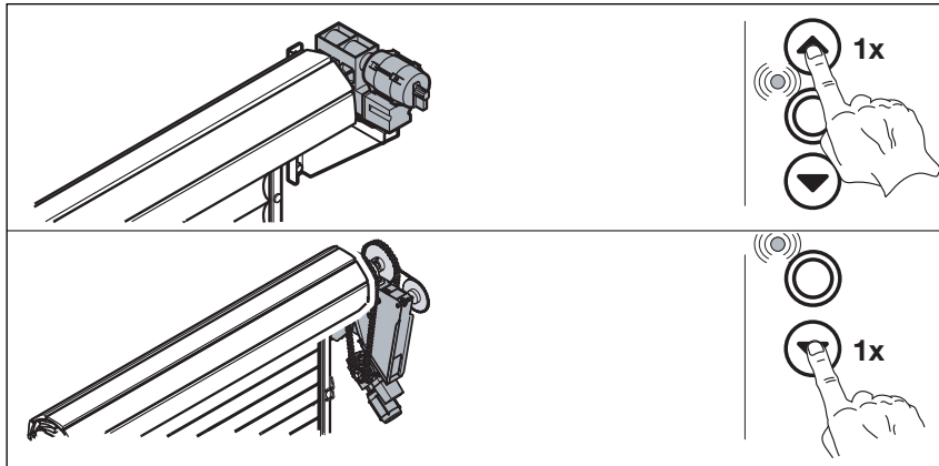
6-2.1 Операция 1: Установите виды монтажа
