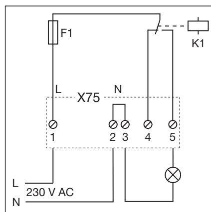
7-4.3 Схема реле и пример подключения для лампы на 230 В
