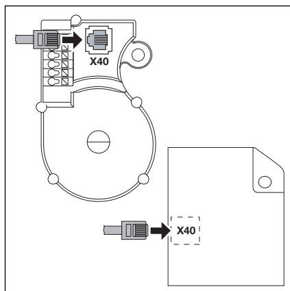
4-2.3 Подсоединение системного провода к - А = датчику положения ворот
