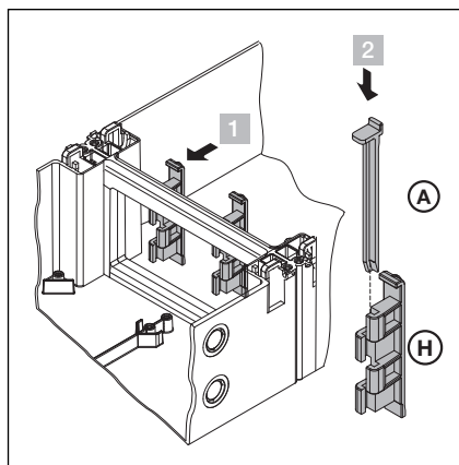
3-3.2 Сборка
