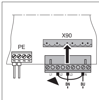
4-6.6 Тип двигателя K09WS: Подключение к сети однофазного переменного тока на X90
