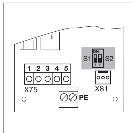
7-4.2 Переключатель режимов работы S1/S2
