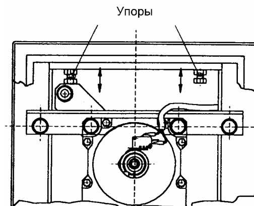
Рис.15 Регулировка упоров.
