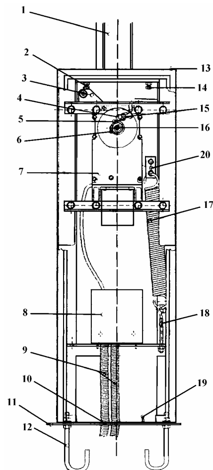
Рис.5 Состав шлагбаума.
